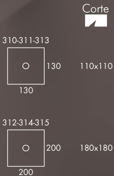
310 1 - Dicróica 50w 311 1 - AR 70 50w 312 1 - Ar 111 50w 313 1 - Par 20 50w 314 1 - Par 30 75w 315 1 - Par 38 90w
