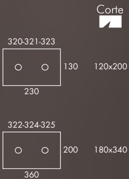
320 2 - Dicróica 50w 321 2 - AR 70 50w 322 2 - Ar 111 50w 323 2 - Par 20 50w 324 2 - Par 30 75w 325 2 - Par 38 90w
