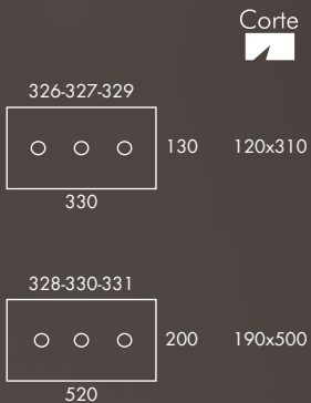
326 3 - Dicróica 50w 327 3 - AR 70 50w 328 3 - Ar 111 50w 329 3 - Par 20 50w 330 3 - Par 30 75w 331 3 - Par 38 90w
