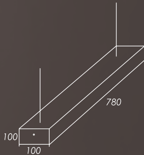
LED 102 - 5 PAR 16 medidas: 780 x 100 x 100
