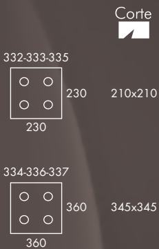
332 4 - Dicróica 50w 333 4 - AR 70 50w 334 4 - Ar 111 50w 335 4 - Par 20 50w 336 4 - Par 30 75w 337 4 - Par 38 90w
