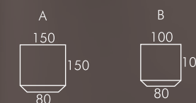
Arandela Externa Alumínio / Vidro temperado Pintado / Escovado 3051 - A - 1 E 27 3051 - B - 1 E 27 ou halopin
